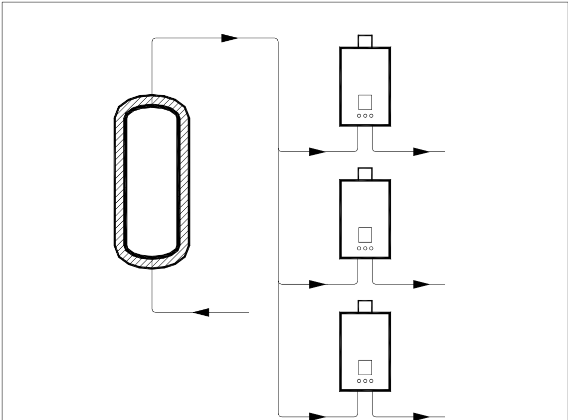
FIG.11 SISTEMA DE ENERGIA AUXILIAR EN LINEA DISTRIBUIDO
