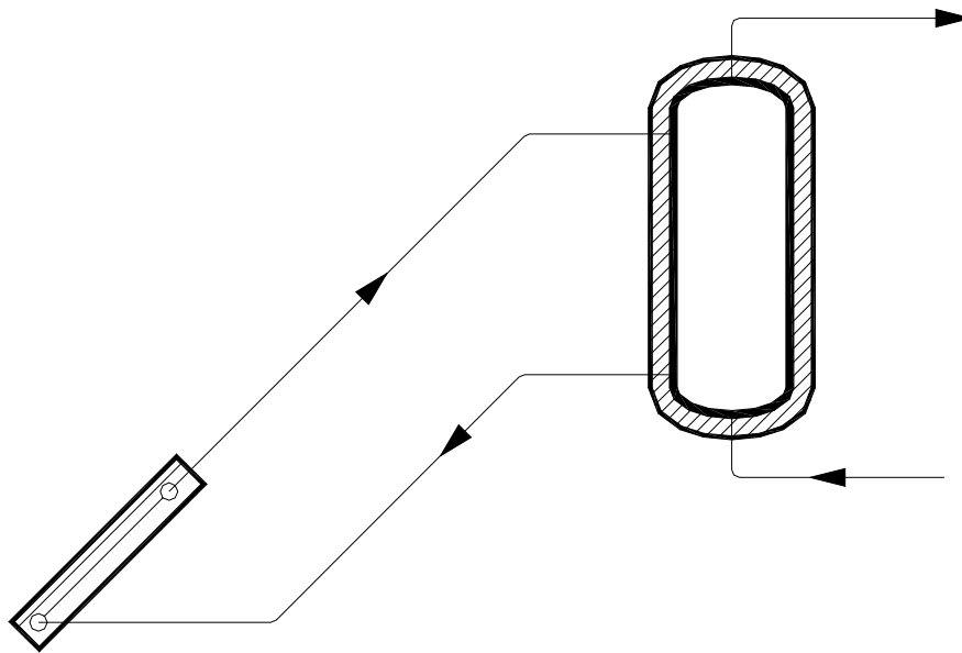
FIG. 1 TERMOSIFON DIRECTO
